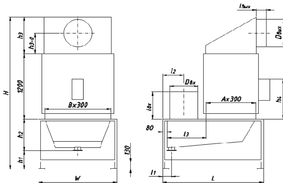
Rys. 1 Podstawowe wymiary multiwirowego hydrofiltra MWF.
