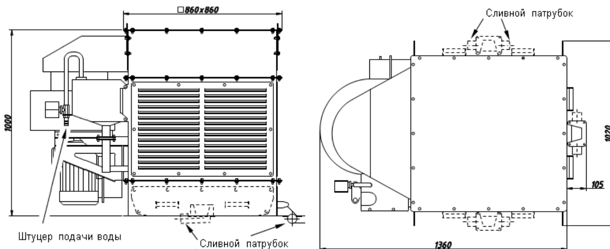
Rys. 2 Podstawowe gabaryty filtra wodnego typu ZONTIK.
