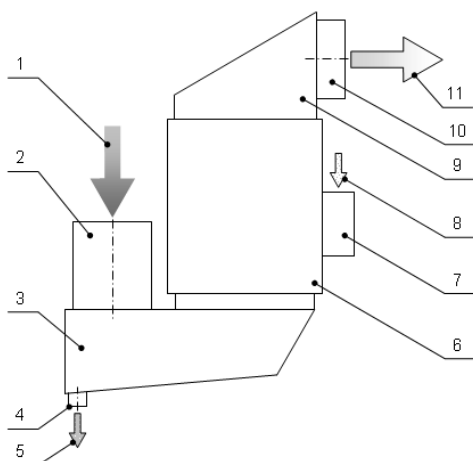
Rys. 1 Ogólny schemat filtra wodnego.
